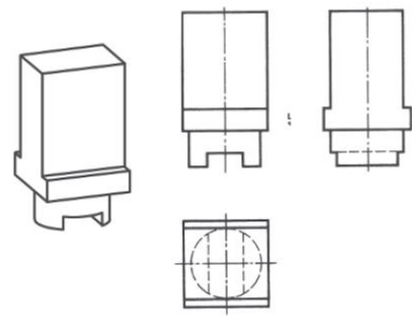
3. Absätze gefräst
