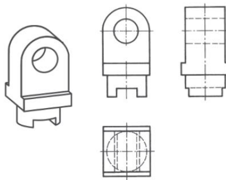
5. Loch gebohrt
