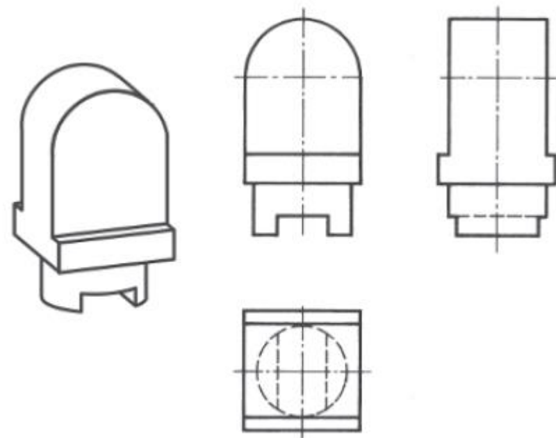
4. Kopf halbrund gefräst
